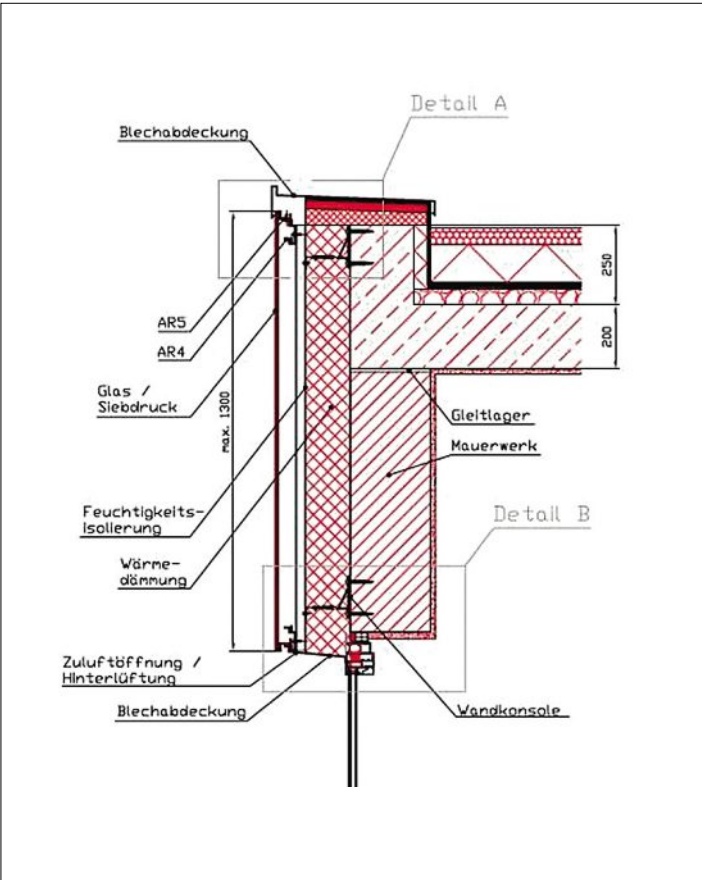
Vertikalschnitt durch den Dachrand.
